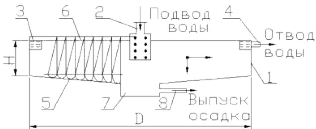
Рисунок 1- Радиальный отстойник
