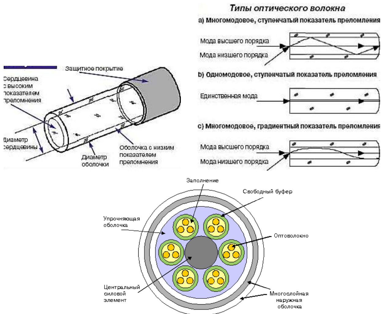
Рисунок 2- Элементы и типы оптических кабелей.
